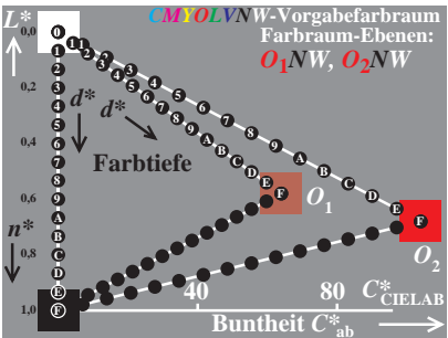
BG090-1, Farbtiefe d^* von O_1, O_2 in (C_{ab}^*, L^*)
