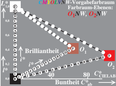
BG091-7, Brilliantheit i^* von O_1, O_2 in (C_{ab}^*, L^*)
