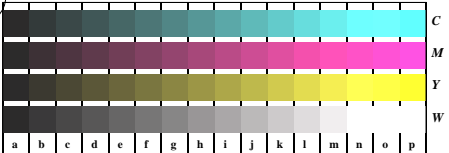
Bild B4n: 16 gleichabständige Stufen W-C, W-M, W-Y und W-N; PS operator LAB* setcolor
