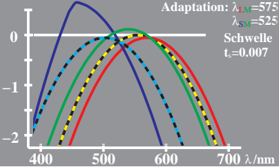
WG060-5, Änderung von LMS beim Farbsehen; Adaptation
