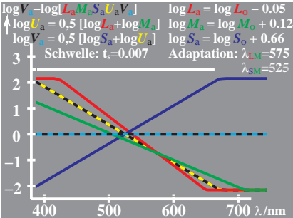
WG061-2, Änderung von LMS beim Farbsehen; Adaptation
