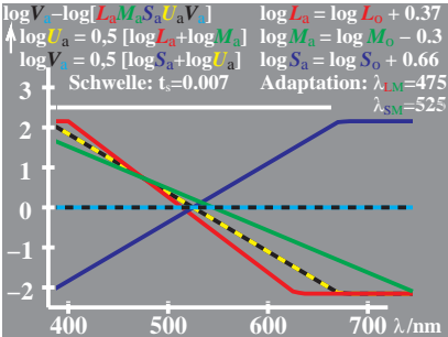
WG061-4, Änderung von LMS beim Farbsehen; Adaptation
