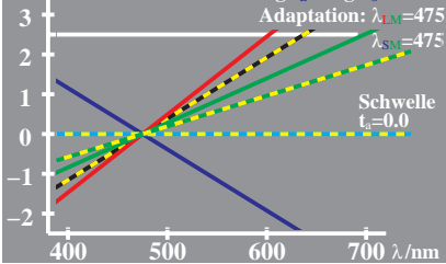
WG280-8, Änderung von LMS beim Farbsehen; Adaptation
