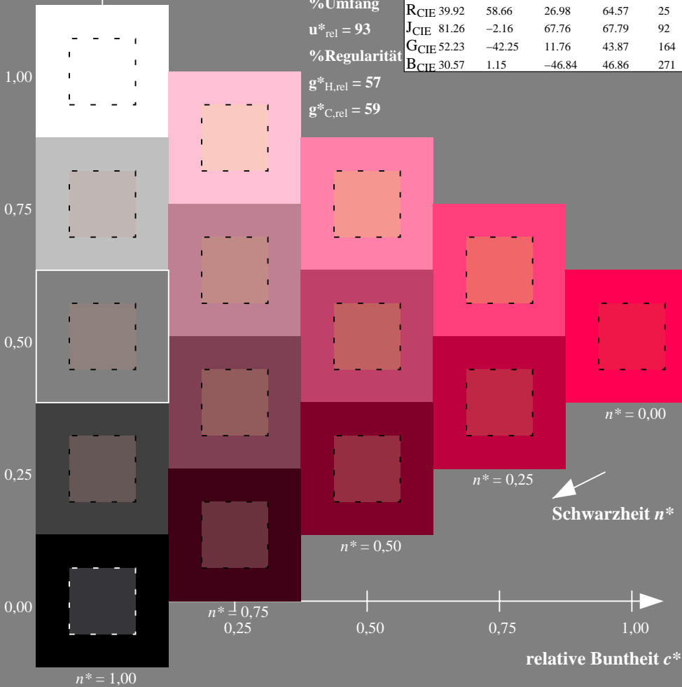
XG620-7, 5stufige Reihen für konstanten CIELAB Buntton 25/360 = 0.069 (links)
