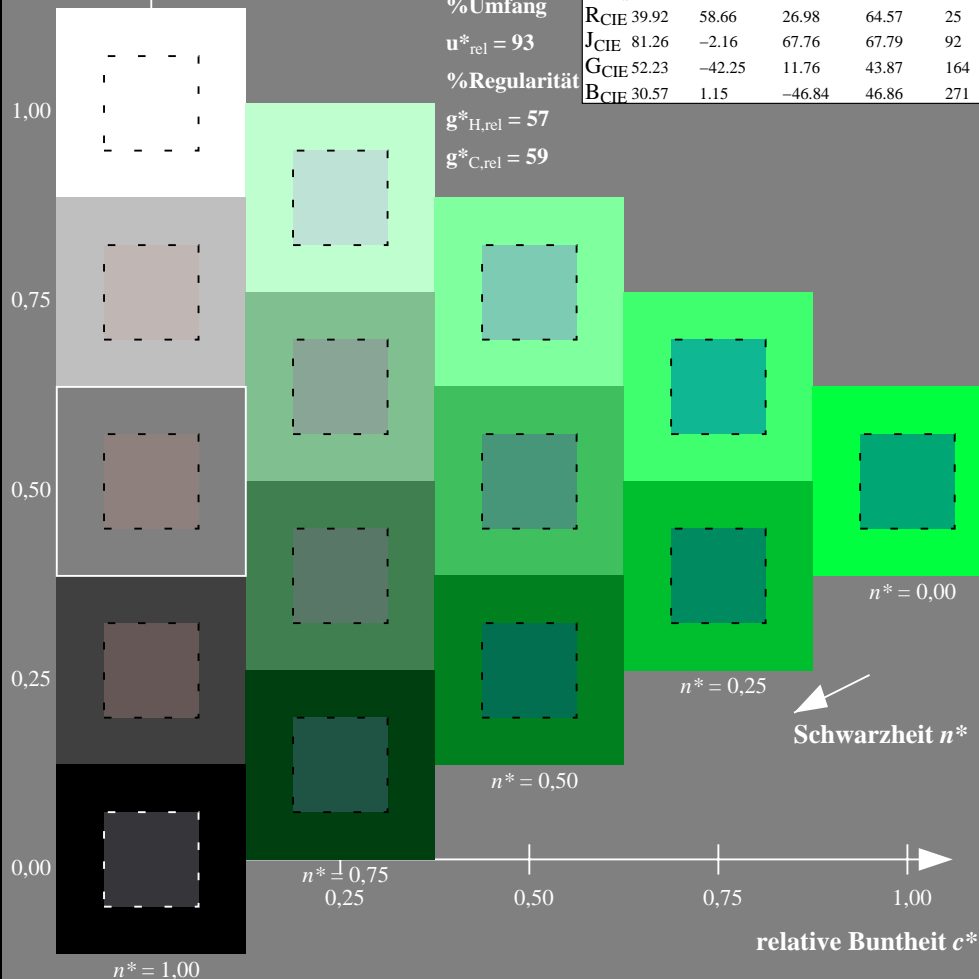
XG620-7, 5stufige Reihen für konstanten CIELAB Buntton 164/360 = 0.457 (links)
