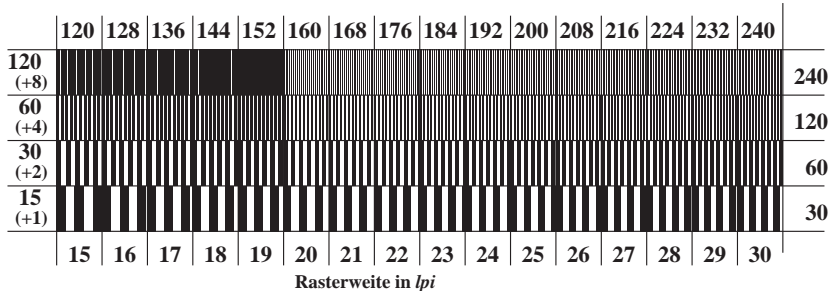
XG761-5, Bild C6: Linienraster unter 90 (oder 0); Benutzung des PS-Operators 000n* setcmykcolor
