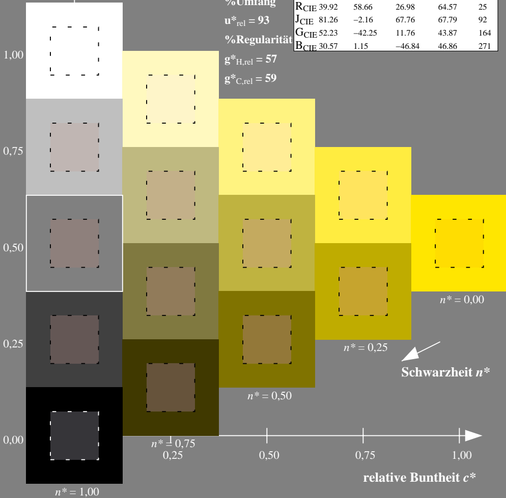
Dg140-7N, 5-stufige Reihen für konstanten CIELAB Bunnton 92/360 = 0,255 (links)
