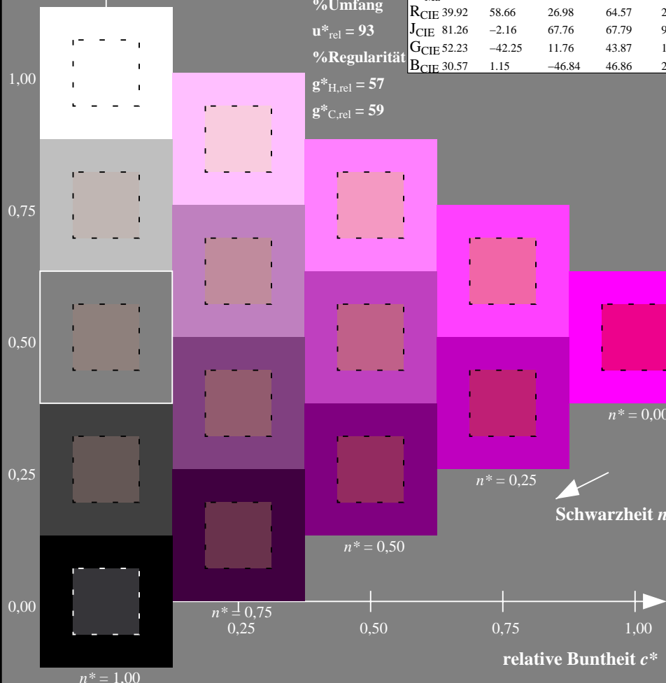
Dg140-7N, 5-stufige Reihen für konstanten CIELAB Bunnton 354/360 = 0.982 (links)
