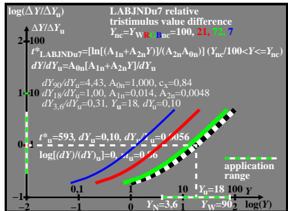
CED70-4A
