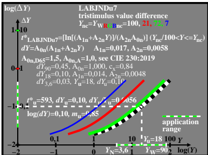
CED70-3A
