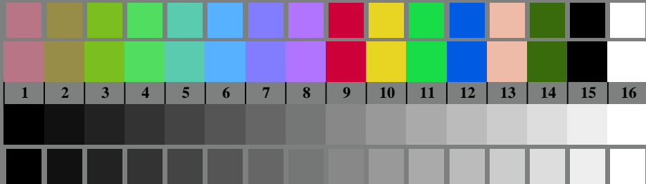
DGE00-7, Bild B3: 14 CIE-Prüffarben nach CIE 13.3 und 16 Graustufen
