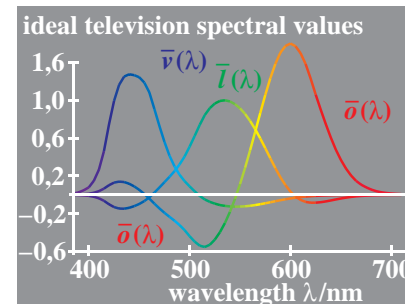
ME211-6, B5_29
