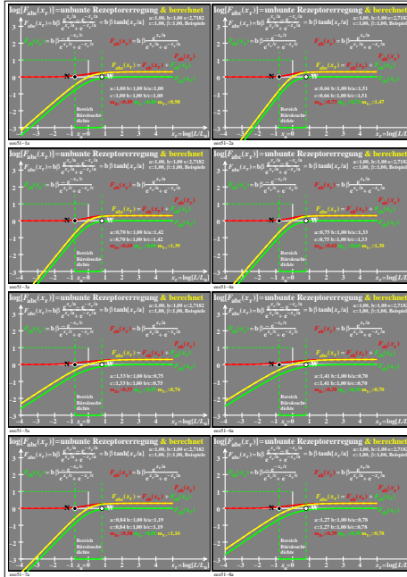
TUB-Prüfvorlage eo5; TUBJND-Modell, Helligkeiten F_{abc} , F_{abc,r} Rezeptorerregungen F_{ab}(R^+) , F_{cb}(G^-) , F_{ab}+F_{cb}(Y^+) (links), relative Erregungen (rechts) für gleiche Parameter a und b
