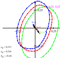
Munsell (Renotation)-Buntheit C = 2 und Helligkeit (Value) V = 1, 5 und 9 in Buntheitsdiagramm ( A_2^*(F,U) , B_2^*(F,U) )
