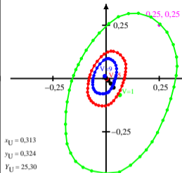
Munsell (Renotation)-Buntheit C = 2 und Helligkeit (Value) V = 1, 5 und 9 in Farbartdiagramm ( a_2(F,U) , b_2(F,U) )
