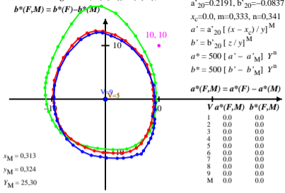
Munsell (Renotation)-Buntheit C = 2 und Helligkeit (Value) V = 1, 5 und 9 in Buntheitsdiagramm ( a^*(F,M) , b^*(F,M) )
