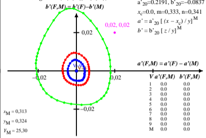
Munsell (Renotation)-Buntheit C = 2 und Helligkeit (Value) V = 1, 5 und 9 in Farbartdiagramm ( a'(F,M) , b'(F,M) )
