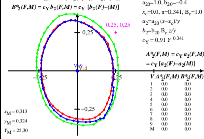
Munsell (Renotation)-Buntheit C = 2 und Helligkeit (Value) V = 1, 5 und 9 in Buntheitsdiagramm ( A_2^*(F,M) , B_2^*(F,M) )
