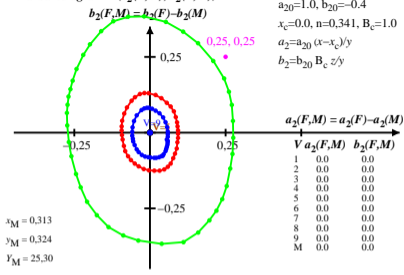
Munsell (Renotation)-Buntheit C = 2 und Helligkeit (Value) V = 1, 5 und 9 in Farbartdiagramm ( a_2(F,M) , b_2(F,M) )
