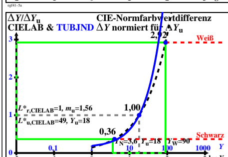
TUB-Prüfvorlage egf4; CIE-Normfarbwertdifferenz \Delta Y/\Delta Y_u = f[\log(Y)] der Farbräume CIELAB & TUBJND, siehe ISO/CIE 11664-4 & CIE 230, viel Information (links), weniger (rechts)
