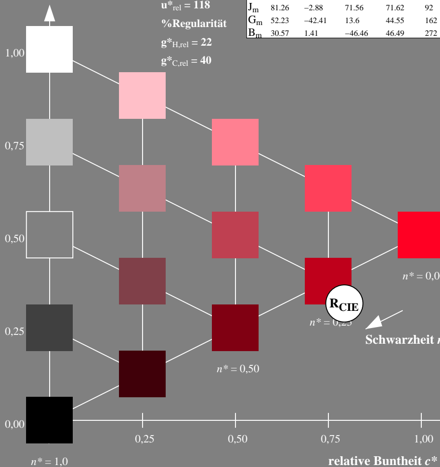
NG260-7, 5 stufige Reihen für konstanten CIELAB Bunnton 25/360 = 0.071 (links)
