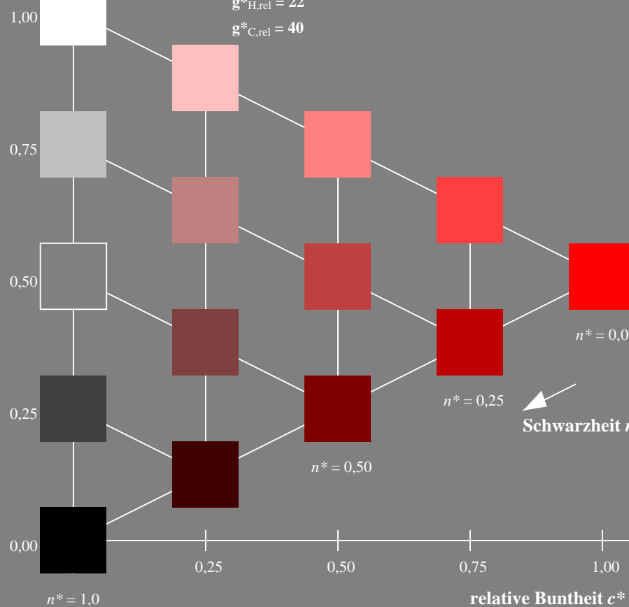
NG260-7, 5 stufige Reihen für konstanten CIELAB Bunton 35/360 = 0.097 (links)
