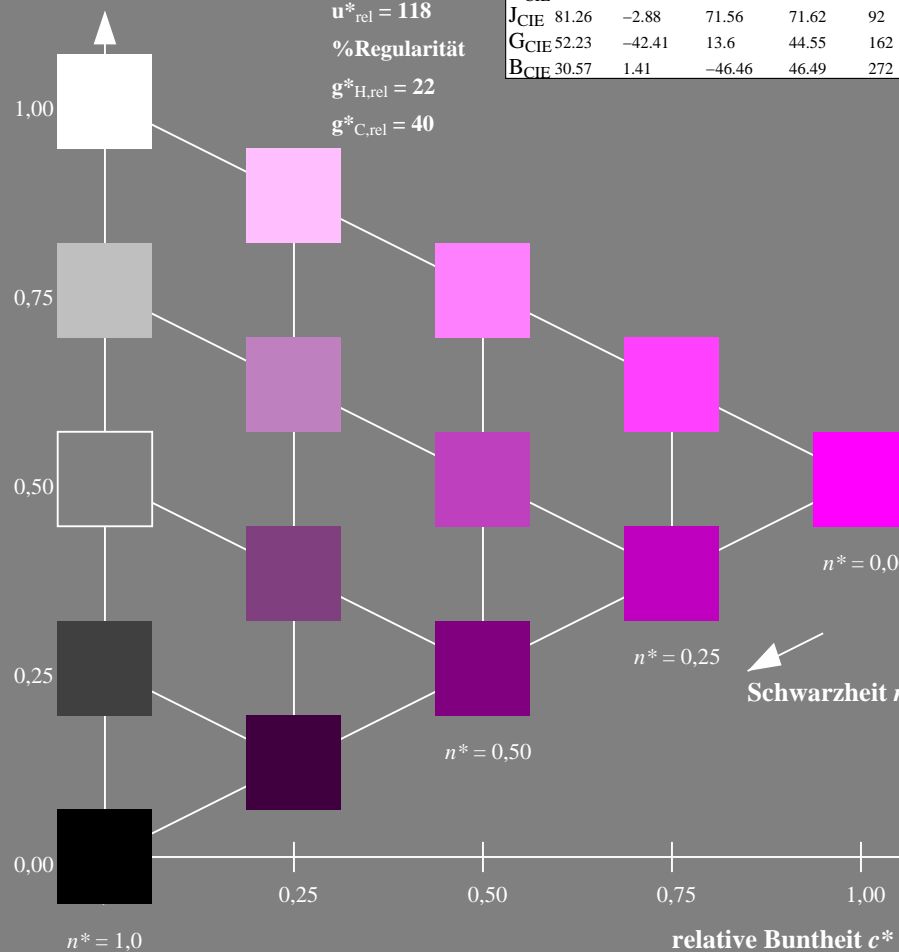
NG260-7, 5 stufige Reihen für konstanten CIELAB Bunton 328/360 = 0.911 (links)
