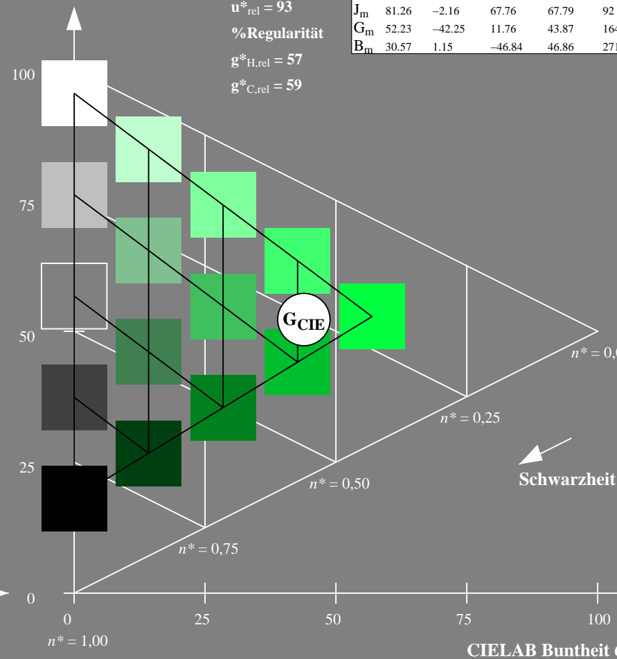
5 stufige Reihen für konstanten CIELAB Bunnton 164/360 = 0.457 (rechts)
