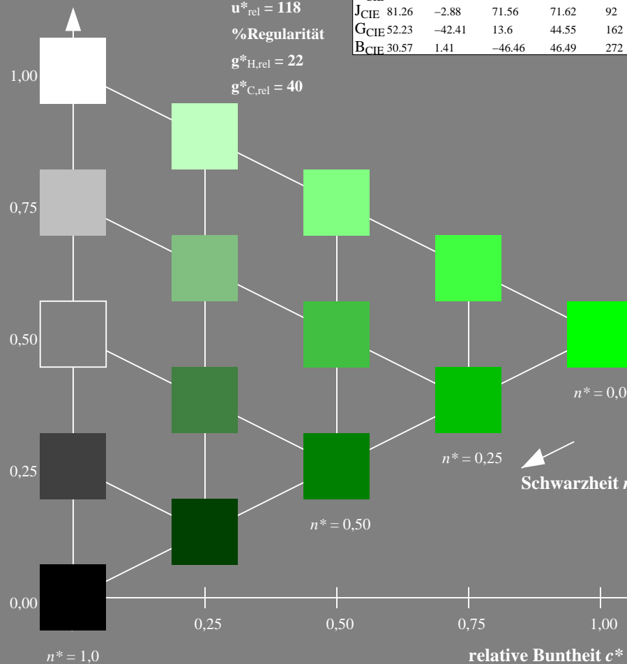
NG260-7, 5 stufige Reihen für konstanten CIELAB Buntton 137/360 = 0.38 (links)
