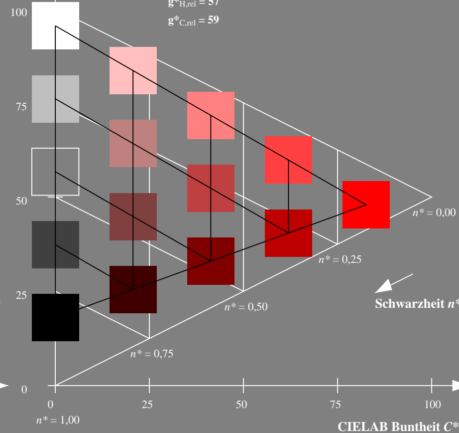
5 stufige Reihen für konstanten CIELAB Bunton 38/360 = 0.105 (rechts)
