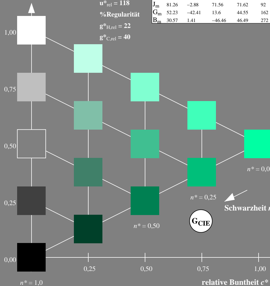
NG260-7, 5 stufige Reihen für konstanten CIELAB Bunnton 162/360 = 0.451 (links)
