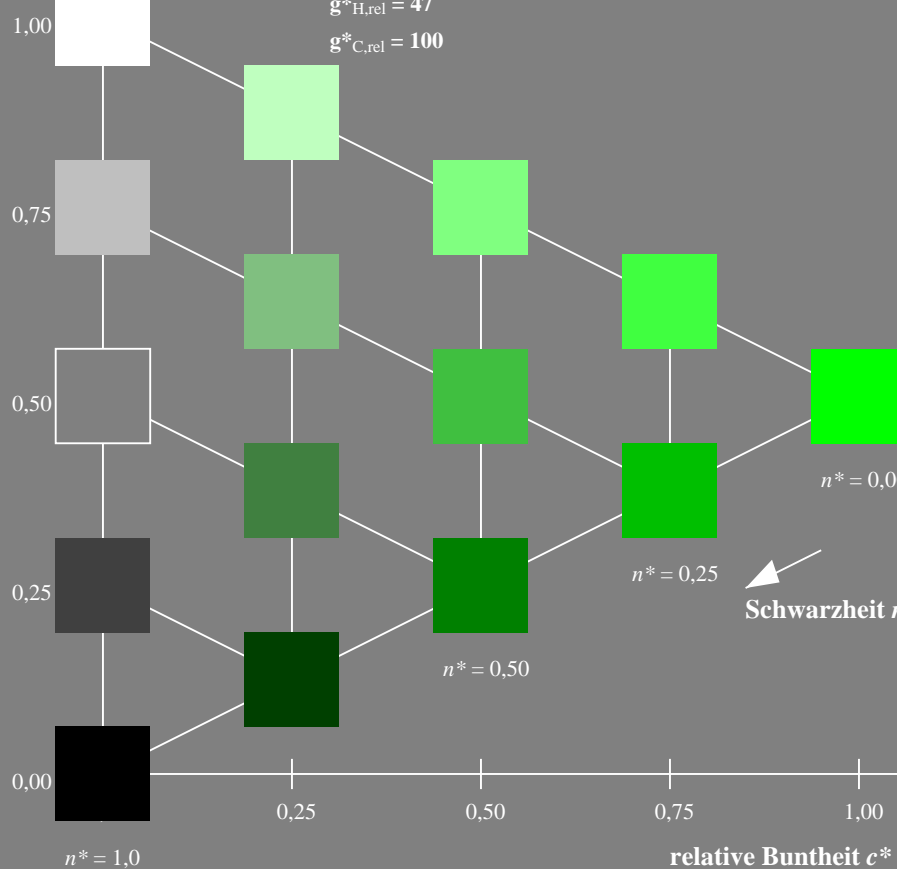
TG270-7, 5 stufige Reihen für konstanten CIELAB Bunnton 167/360 = 0.464 (links)
