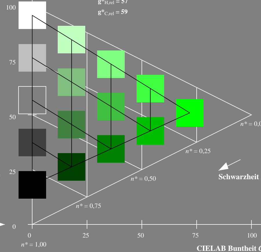
5 stufige Reihen für konstanten CIELAB Bunnton 151/360 = 0.419 (rechts)
