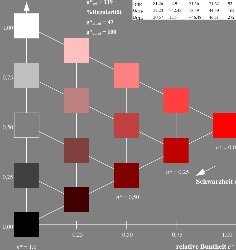
TG270-7, 5 stufige Reihen für konstanten CIELAB Bunnton 24/360 = 0.067 (links)
