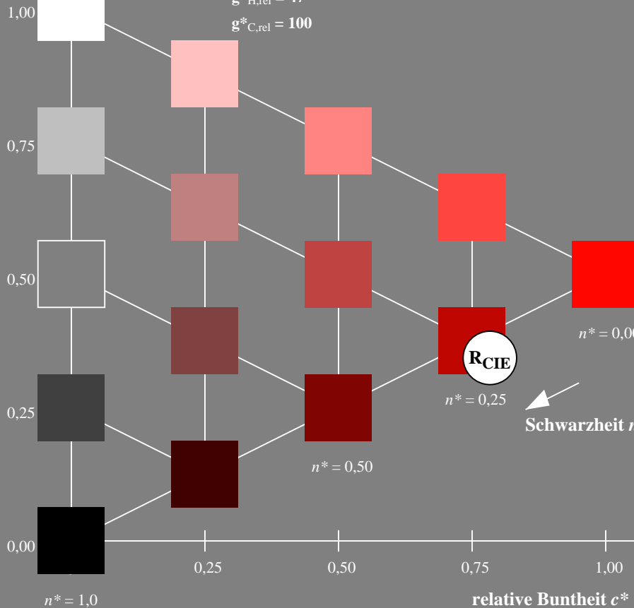
TG270-7, 5 stufige Reihen für konstanten CIELAB Buntton 25/360 = 0.071 (links)
