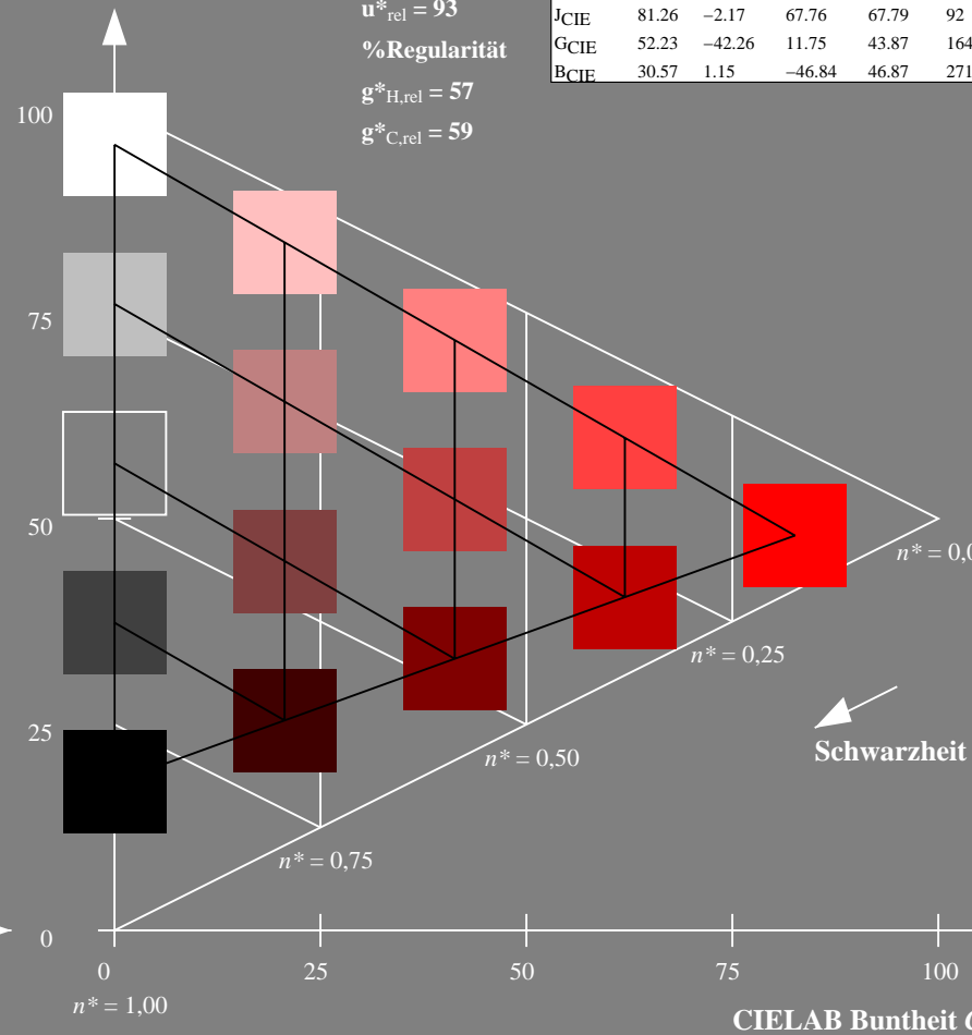
5 stufige Reihen für konstanten CIELAB Bunnton 38/360 = 0.105 (rechts)
