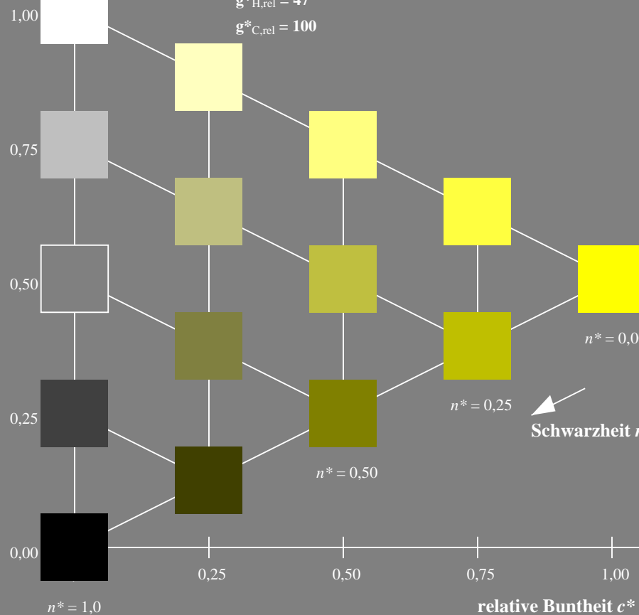
TG270-7, 5 stufige Reihen für konstanten CIELAB Buntton 91/360 = 0.253 (links)
