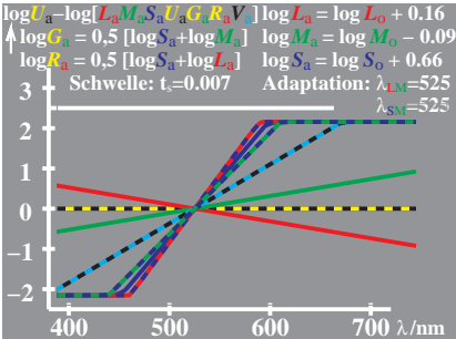
WG081-4, Änderung von LMS beim Farbsehen; Adaptation
