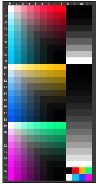
AF560-71 La partie de graphique AF56 de test avec 1080 couleurs; paliers de 9 ou 16 couleurs; les données de la colonne (b-m): rgb 3-110110-L0 cmy6*
