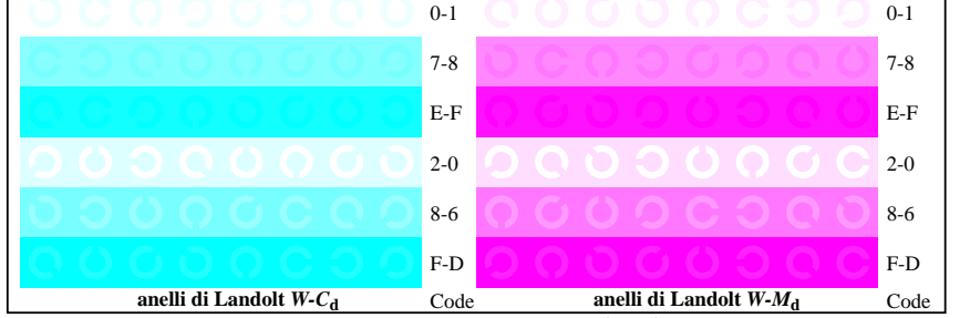
AI281-5, Fig. B6Wdd: anelli di Landolt W-C d ; W-M d ; PS operator: rgb->rgb dd setrgbcolor
