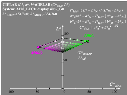
grafico TUB-AI78; Esempi di metriche di colori CIE dati di elementari colori e di uscita sui dispositivi
