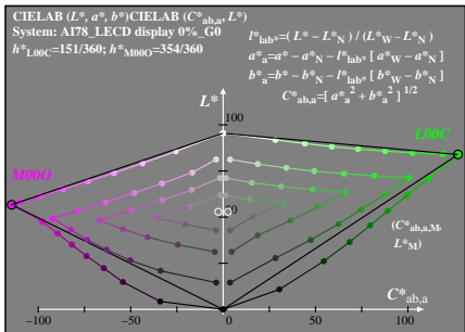
grafico TUB-AI78; Esempi di metriche di colori CIE dati di elementari colori e di uscita sui dispositivi
