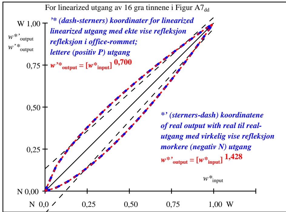
artikkelen 2, AN591-3dd: 01042
