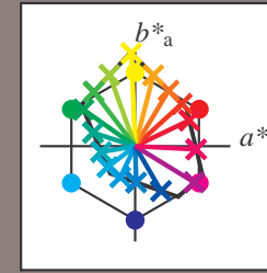
FRS15_90aM; adaptierte CIELAB-Daten
