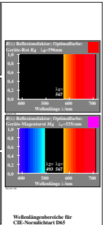
Wellenlängenbereiche für CIE-Normlichtart D65
