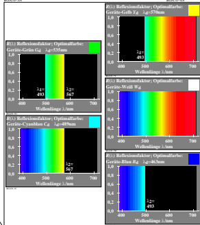
Wellenlängenbereiche für CIE-Normlichtart D65
