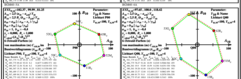
BGM60-7A, BGM60-8A
