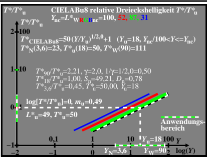
BGX81-2A
