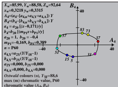
CE211-6A_1
