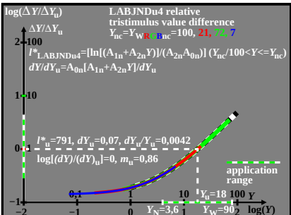
CEC40-4A
