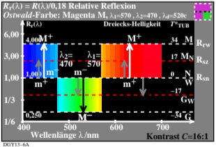
DGY13-6A
