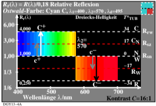
DGY13-4A
