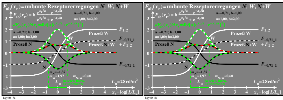
TUB-Prüfvorlage hgy6; Modell für Erregungsfunktionen F_{ab}(x_r) , Prozesse N, W, N+W und Ableitungen Tangens hyperbolicus \tanh(x_r) & modifiziert mit e^{\pm x_r/a} und 10^{\pm x_r/a} ; a=-0,71 & 1,00 ; a' = a \ln(10)
